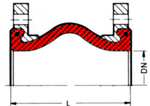
Megjegyzés | gumikompenzátor - A1-es típus | 3D méreterajz
