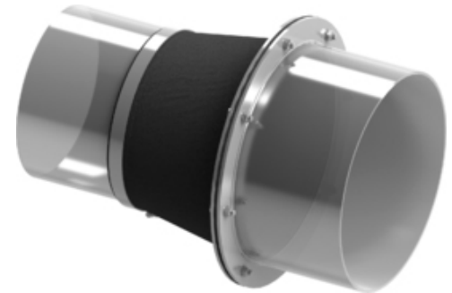
Megjegyzés | szövetkompenzátor - 52-es típus | 3D nézet
